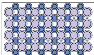
Beispiel: Interaktiver Taschenfederkern mit unterschiedlich großen Spiralfedern auf gleicher Fläche = 58 Federn
